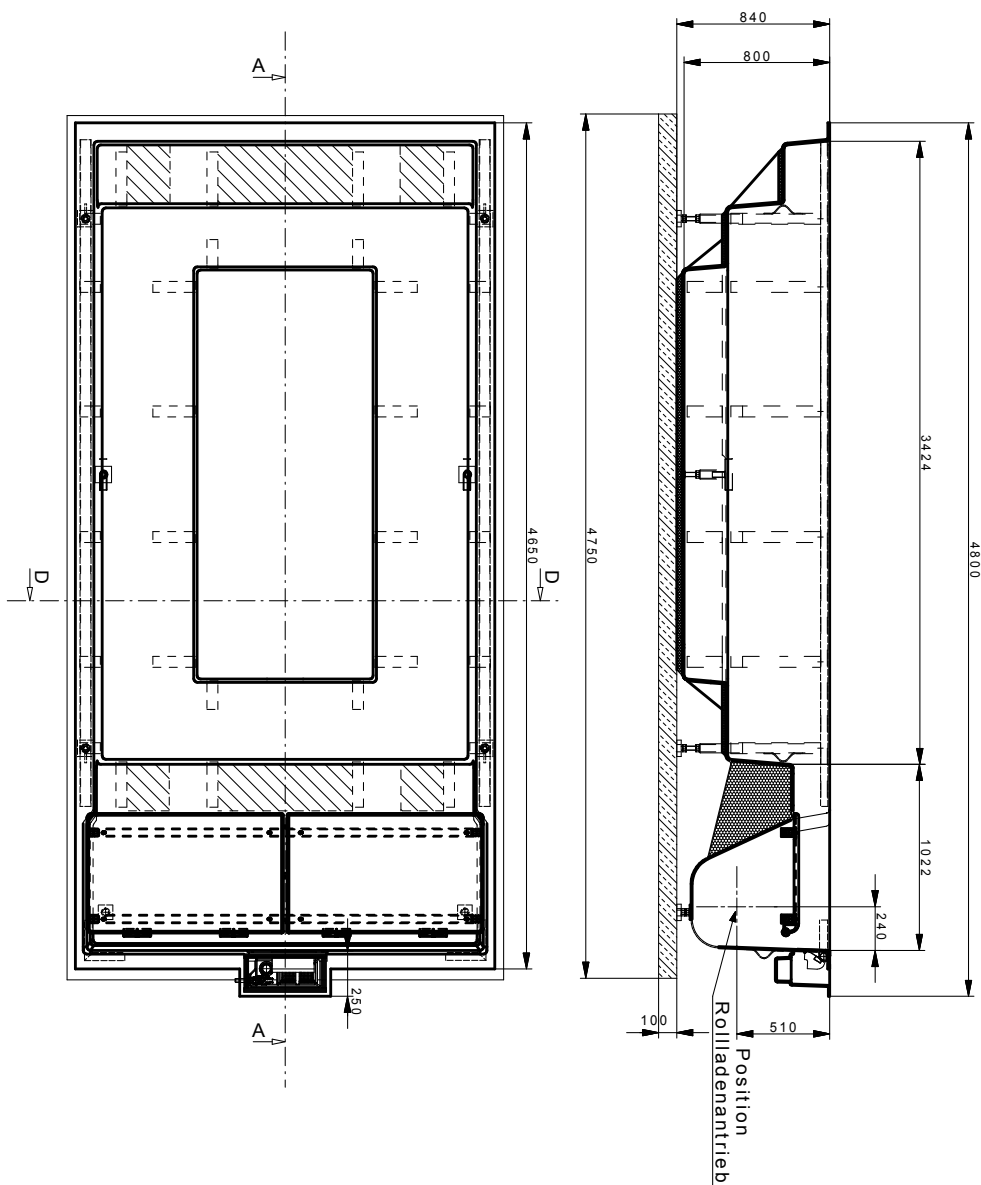
Schnitt A - A
