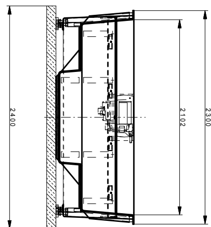
Schnitt D - D
